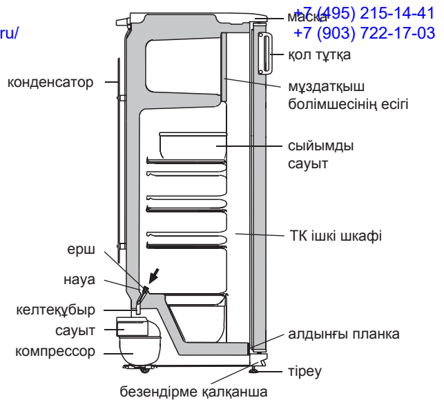
4 сурет — Еріген суды ТК-нан ағызу схемасы
